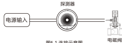
图5.1 连接示意图
