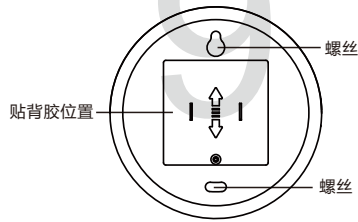
图4.2 安装示意图
