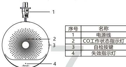
图3.1 外观示意图
